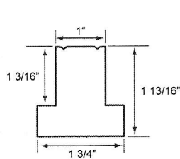
T-POST
