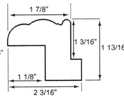
MALIBU Z-FRAME
