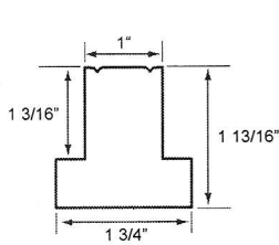
T-POST
