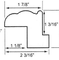
MALIBU Z-FRAME
